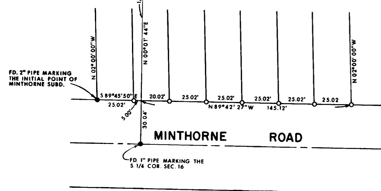
DETAIL SCALE: 1" = 30'
