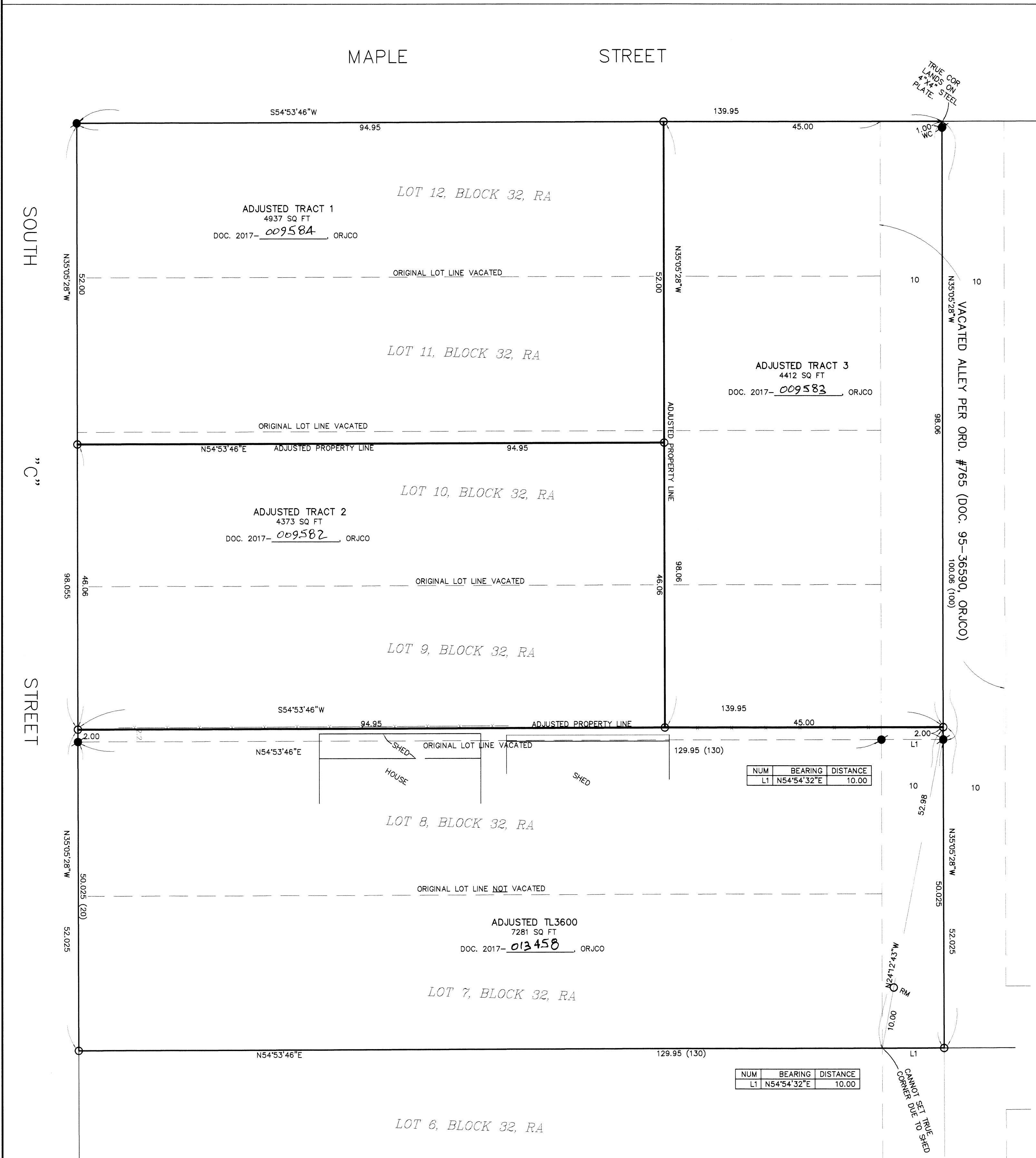
ENLARGEMENT - 1"=10'
